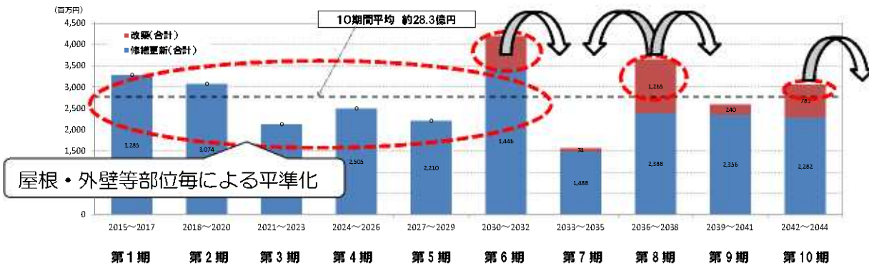
図1 10期間の平準化前の工事費
