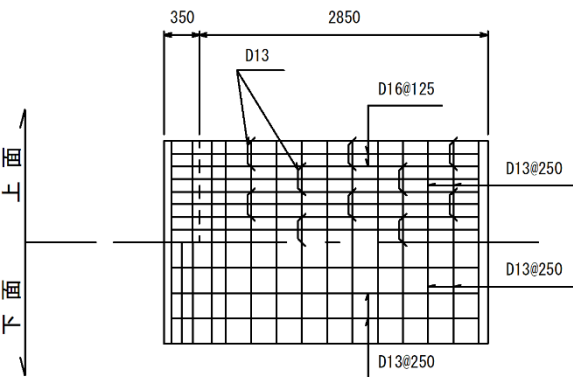
底版配筋図
