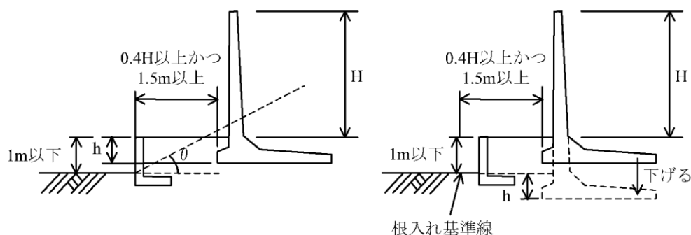
図 5-9 上部・下部擁壁を近接して設置する場合 (その 3)
