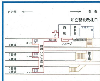
今年度を実施する工事の完成平面図
