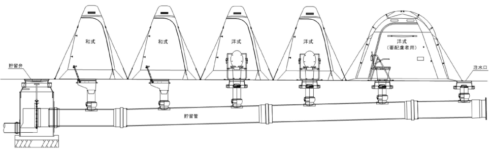
マンホールトイレ構造図 S=Free
