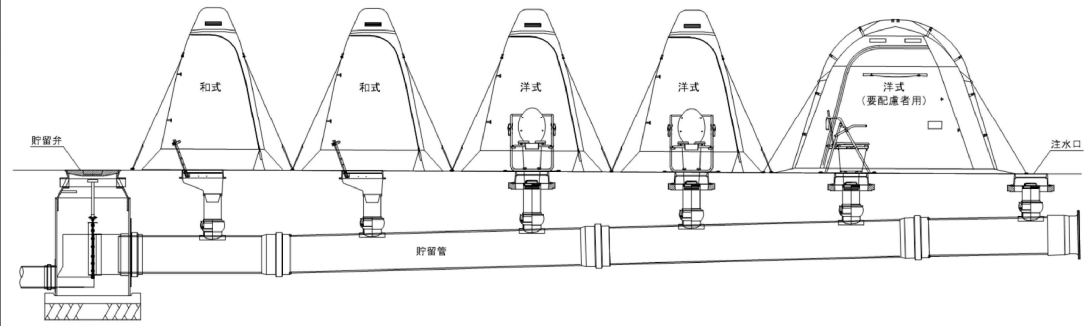
マンホールトイレ構造図 S=Free
