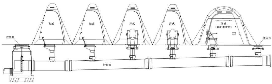
マンホールトイレ構造図 S=Free
