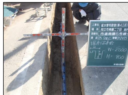
配水管布設 ポリエチレン管
