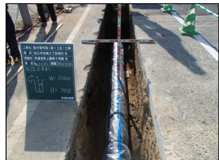
配水管布設 鋳鉄管
